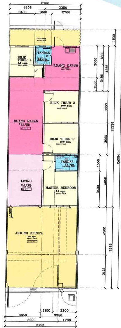
RUMAH TERES 1 TINGKAT ( 22' x 80' )
