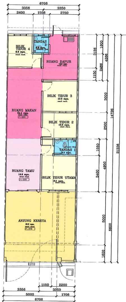
RUMAH TERES 1 TINGKAT ( 22' x 70' )
